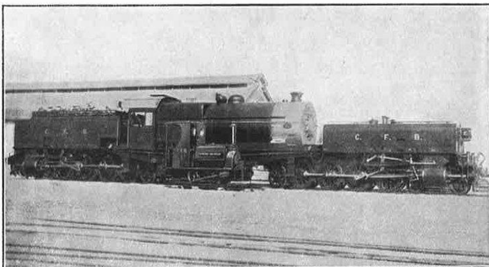
A GRANDE LOCOMOTIVA GARRATT CONSTRUÍDA NAS OFFICINAS DE BEYER PEACOCK & Co., LTD., E A PRIMEIRA QUE FEZ SERVIÇO NA LINHA.
