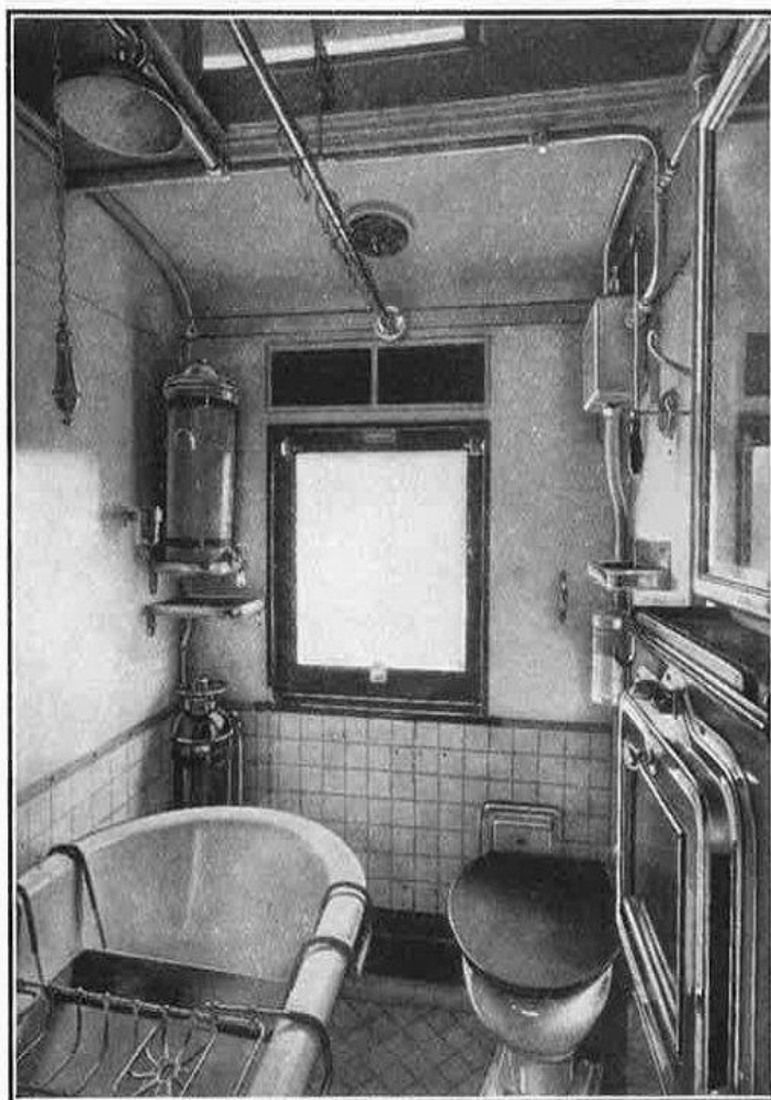
CASA DE BANHO, CONSTRUÍDO PELA METROPOLITAN-CAMMELL CARRIAGE WAGON AND FINANCE Co., LTD., BIRMINGHAM.
