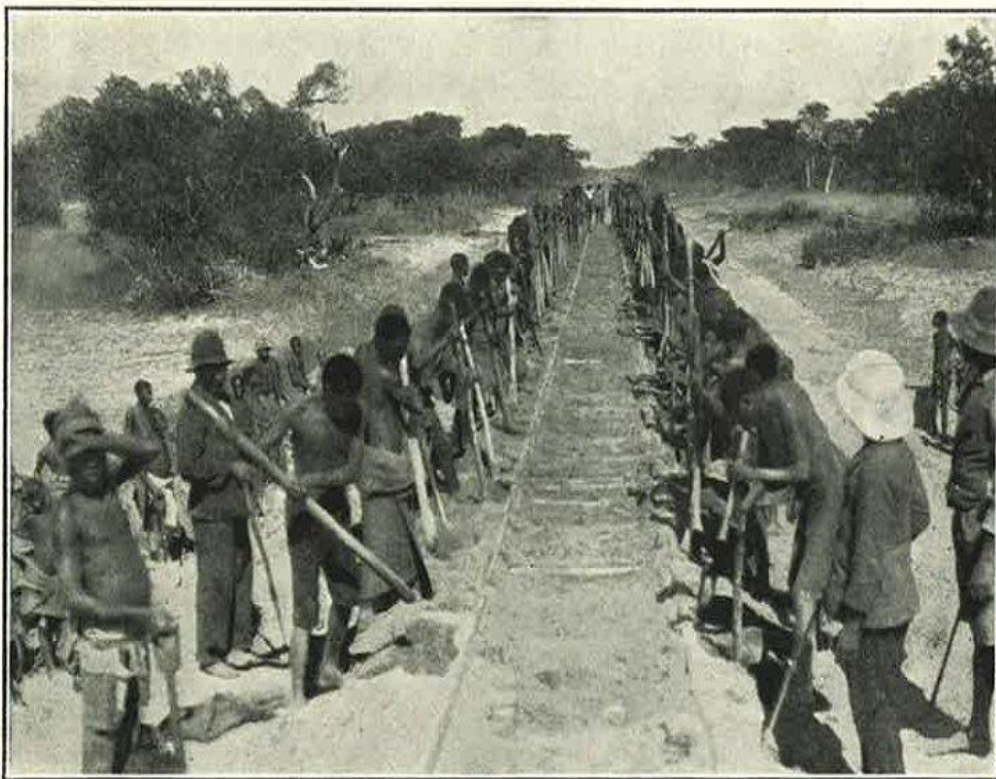
ASSENTAMENTO DE LINHA. TRABALHADORES ATACANDO OS CARRIS E AS TRAVESSAS.
