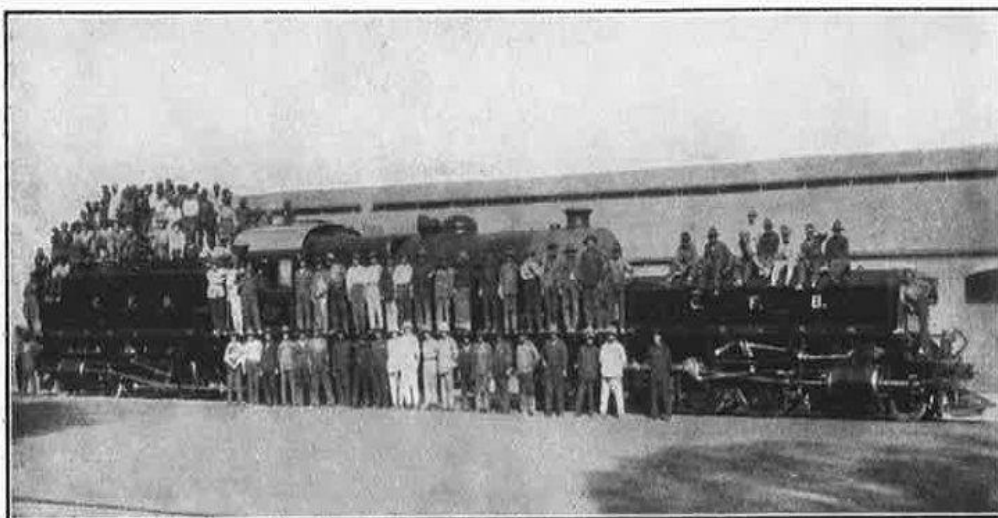
LOCOMOTIVA GARRATT. ESTAS MACHINAS SÃO AS MAIS PODEROSAS QUE EXISTEM PARA UMA LINHA DA BITOLADE 1M06 E CARRIS DE 30 KILOS. PODEM REBOCAR 500 TONELADAS NAS PARTES MAIS DIFFICEIS DA LINHA.
